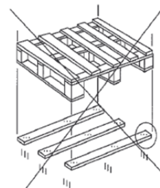
Palet cu grinzi longitudinale pe toate părțile – 3 scânduri inferioare suplimentare așezate prin partea de jos, conform imaginii
